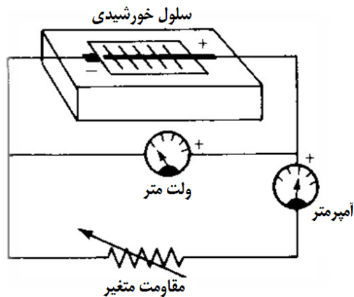
شکل ۲. طرح‌واره مدار واحد اندازه‌گیری پارامترهای عملکردی پنل.
