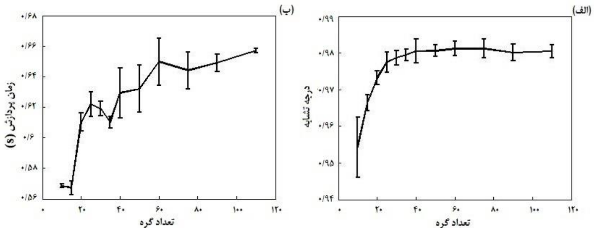
شکل ۷. الف) درجه تشابه تصویر منحنی بازسازی شده با تصویر اصلی، ب) زمان لازم برای پردازش الگوریتم در نرم‌افزار MATLAB (مقادیر میانگین بدست آمده از تحلیل تصاویر سه رقم فایر، فانتسیا و سانته).
