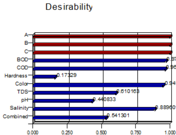
شکل ۱۱- سطوح پاسخ درصد تغییرات BOD, COD, pH, Hardness, color, TDS and Salinity بر مبنای تکرار و ضخامت فیلتراسیون
