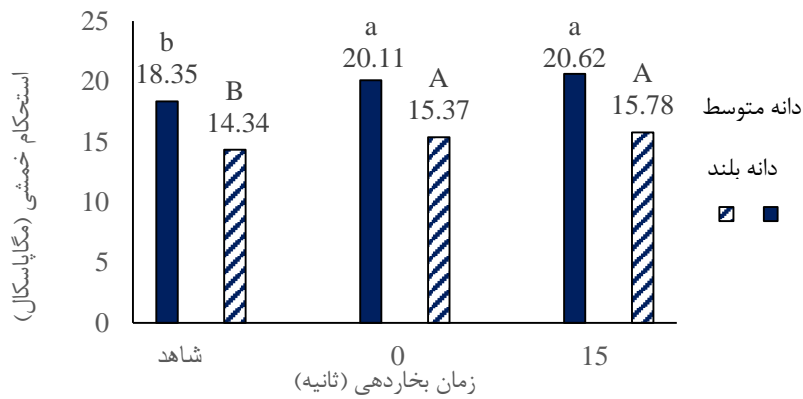
شکل ۴- استحکام خمشی در مدت زمان بخاردهی
