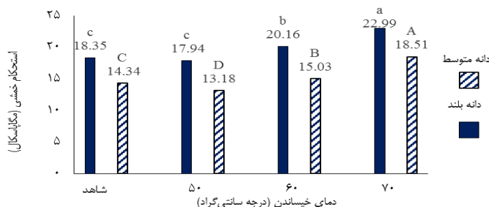
شکل ۲- استحکام خمشی در دماهای مختلف خیساندن
