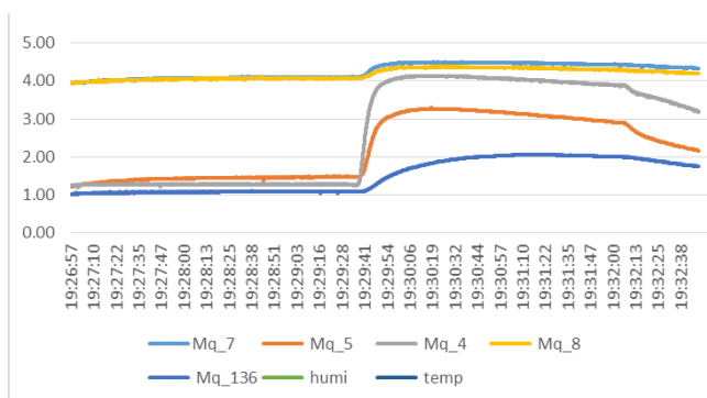
شکل ۱- نمودار سامانه ماشین بویایی (سمت چپ)، سیگنال خروجی آرایه حسگری (سمت راست)
