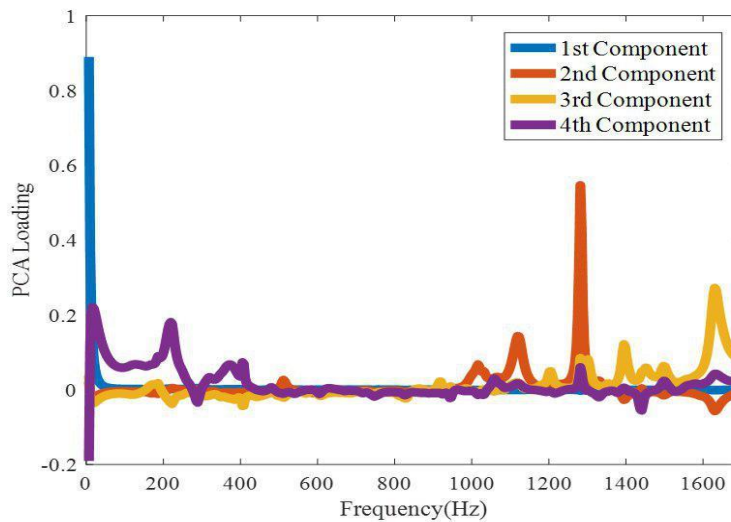
شکل ۵- آنالیز مؤلفه ی اصلی صدای زنبورهای عسل.
