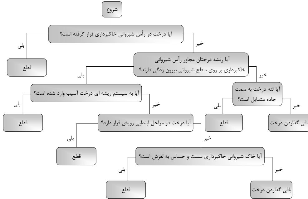
شکل ۶- مدل چارتی یا توصیفی برای تعیین عرض حریم بهینه جاده‌های جنگلی
