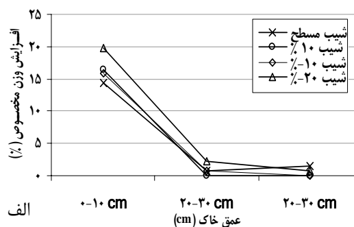
شکل ۶- تغییرات وزن مخصوص ظاهری در عمق‌های مختلف با توجه به شیب مسیر (الف)، مقایسه میانگین وزن مخصوص قبل و بعد از تردد (آزمون دانکن) (ب)، (حروف لاتین نامتشابه بیانگر معنی‌دار بودن اختلاف میانگین‌ها در سطح احتمال ۹۵ درصد است)
