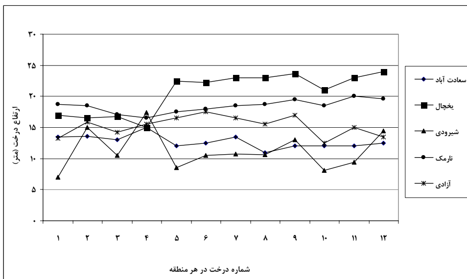
شکل ۲- پراکنش ارتفاع درختان مطالعاتی در پنج منطقه
