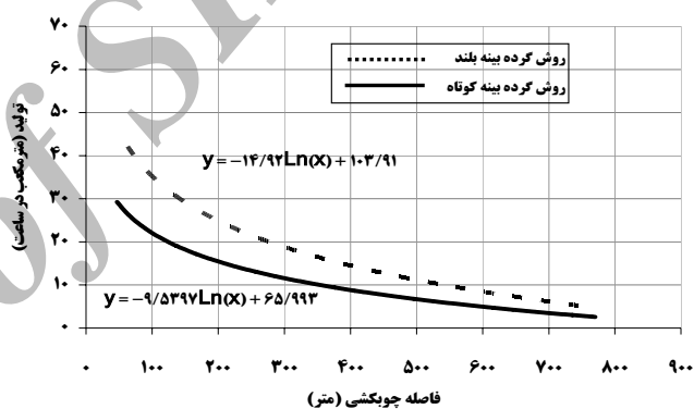
شکل ۳- تغییرات تولید چوبکشی در دو روش گرده‌بینه کوتاه و بلند در ارتباط با فاصله حمل
