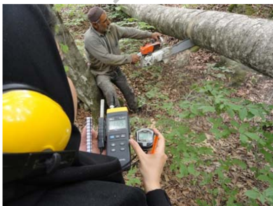
شکل ۱- اندازه‌گیری شدت صدا با دستگاه صداسنج
