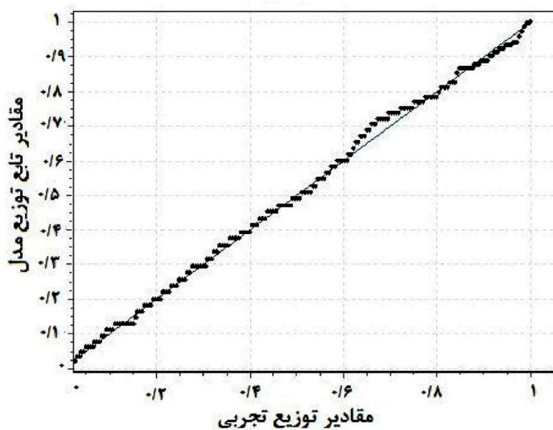
شکل ۱- نمودار P-P توزیع بتا
