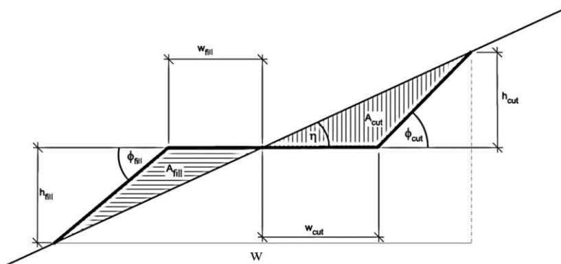
شکل ۳- اجزای مقطع عرضی استاندارد جاده‌های جنگلی. W عرض ساختمانی جاده؛ A_{cut} سطح خاک‌برداری؛ A_{fill} سطح خاک‌ریزی؛ \phi_{fill} شیب ترانشه خاک‌ریزی؛ \phi_{cut} شیب ترانشه خاک‌برداری؛ \eta شیب زمین؛ W_{cut} عرض خاک‌برداری؛ W_{fill} عرض خاک‌ریزی؛ h_{cut} ارتفاع خاک‌برداری؛ W_{fill} ارتفاع خاک‌ریزی (Stuckelberger et al., 2006).
