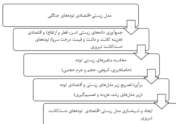
شکل ۳- روندنمای پژوهش
