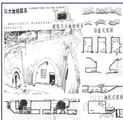
تصاویر ۳ و ۴. خانه‌های زیرزمینی منطقه loess در شمال چین، خانه به صورت گروهی در شکل‌های مختلف در اطراف یک حیاط قرار گرفته‌اند و با یک رامپ به سطح زمین متصل می‌شوند. در این منطقه نوع بازشوها متفاوت است و بازشوها بزرگ‌تر و متعددتر می‌باشند. حیاط با تمام المان‌های خود در پایین‌تر از سطح زمین قرار گرفته‌اند. مأخذ: Crouch, ohnson, 2001: 72
