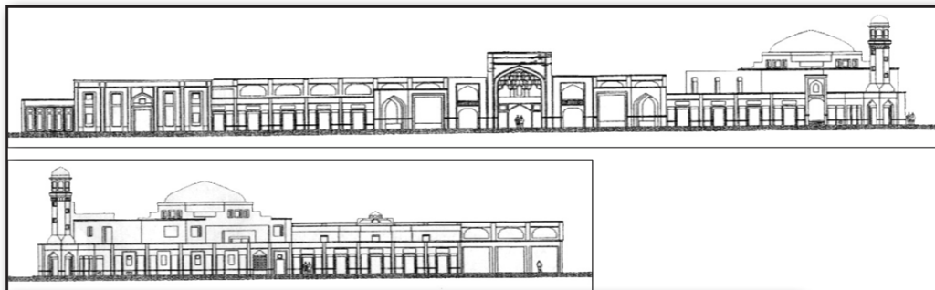
تصویر ۲۷. دید از بیرون به سردر و میدان جدید عالی قاپو (بالا: نمای شمالی) - (پایین: نمای غربی). مأخذ: رضازاده و همکاران، ۱۳۷۸ Fig 27. North and west elevations of the complex . Source :Rezazadeh et al, 1999.
