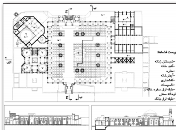
تصویر ۲۶. پلان طراحی جدید طبقه اول میدان و سردر عالی قاپو، نما و برش ب-ب، نما و برش ج-ج. مأخذ: رضازاده و همکاران، ۱۳۷۸. Fig 26. Plan view of the first level of the final concept, section B-B and Section C-C. Source: Rezazadeh et al, 1999.
