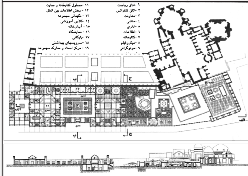
تصویر ۲۸. پلان طبقه همکف سایت باستان‌شناسی و مجموعه فرهنگی، برش الف-الف. مأخذ: رضازاده و همکاران، ۱۳۷۸. Fig 28. Plan view of ground level of the excavation area and the cultural complex . Source: Rezazadeh et al, 1999.
