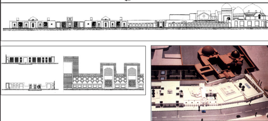
تصویر ۲۹. پلان زیرزمین سایت باستان‌شناسی و مجموعه فرهنگی، نمای غربی (تصویر بالا)، نمای غربی (تصویر وسط) نما برش ب-ب، ج-ج و جزئیات نما (تصویر پایین سمت چپ). مأخذ: رضازاده و همکاران، ۱۳۷۸، ماکت سایت باستان‌شناسی (تصویر پایین سمت راست). مأخذ: آرشیو رضازاده. Fig 29. Underground of excavation area, plan view, west elevation, section B-B, section C-C . Source :Rezazadeh et al, 1999. Model of archaeology area. Source : Archive of Rezazadeh.
