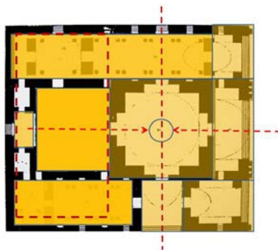
تصویر ۹. جانمایی اندامها در سروستان (پایین) و فیروزآباد (بالا). مأخذ: پیرنیا، ۱۳۸۲. Fig.9. Space organization in Sarvestan and Firooz Abad palaces. Source: Pirniya, 2003.
