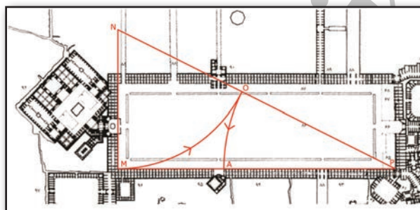
تصویر ۶. تقسیم ضلع میدان به نسبت طلایی به وسیله جلوخان ورودی مسجد شیخ لطف‌الله. مأخذ: اردلان و بختیار، ۱۳۹۰.
