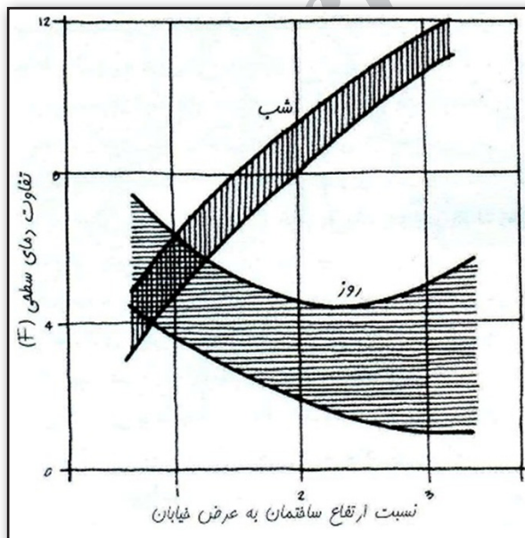
نمودار ۱. اثر برش عرضی خیابان شمالی-جنوبی بر دمای سطحی. مأخذ: Ahmed, 1994: 48. Diagram 1. Effect of north-south street section on surface temperature. Source: Ahmed, 1994: 48
