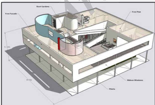
تصویر ۳. سه بُعدی ویلا ساووی، ۱۹۲۸-۱۹۳۰، لوکوربوزیه، فرانسه، پولسی، مأخذ: www.caad2.asro.kl.euven.b
