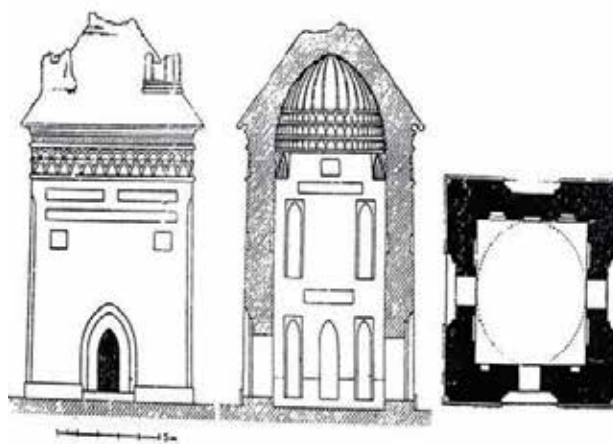
تصویر ۵. پلان، برش و نماهای مقبره متبرکه شمس آل رسول، آمل. مأخذ: www.Arthut.com.
