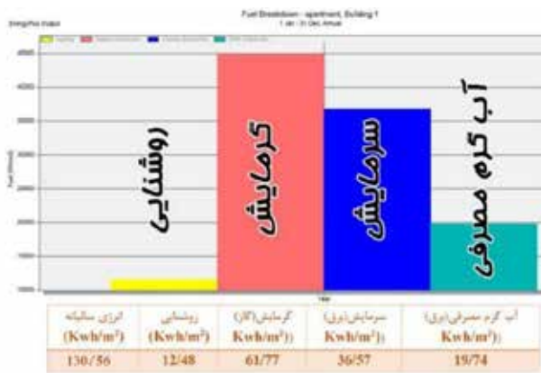
تصویر ۱۵. انرژی مصرفی در بخش‌های مختلف گزینه پیشنهادی، در شرایطی مشابه با شرایط طرح مصوب. مأخذ: نگارندگان.
