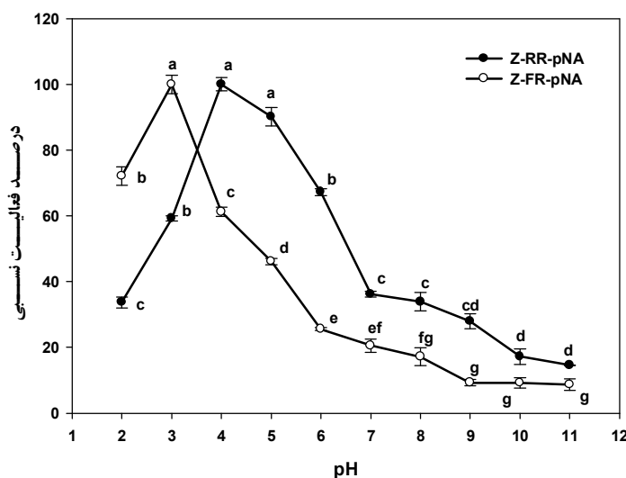
(نمودار ۵) - فعالیت پروتئینازی عصاره اووسیت سن سبز پسته در pH های مختلف
