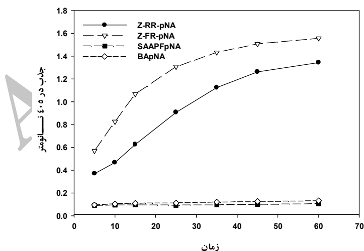
نمودار ۳- فعالیت هیدرولیتیک عصاره اووسیت سن سبز پسته روی سوبستراهای ویژه پروتئینازی
