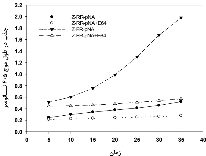
(نمودار ۹) - اثر مهارکننده E-64 بر فعالیت هیدرولیتیک عصاره اووسیت و سن سبز پسته
