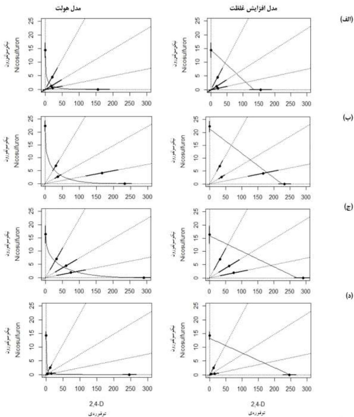
شکل ۳- نمودارهای آیزوبول (هم‌اثر) لجستیک لگاریتمی سه پارامتره برای اثر اختلاط توفوردی آمین با نیکوسولفورون در آب دیونیزه (الف)، محتوی کلرور کلسیم (ب)، کلرور منیزیم (ج) و کلرور آهن III (د) بر زیست توده علف هرز گاوپنبه با برازش مدل افزایش غلظت (راست) و مدل هولت (چپ) می‌باشد.
