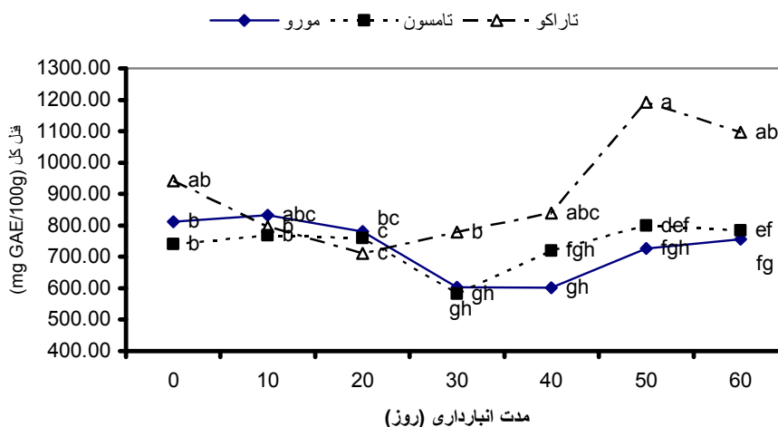
شکل ۶- تغییرات فنل کل میوه پرتقال تاسون، تاراگو و مورو پس از ۶۰ روز در دمای ۷ درجه سانتی گراد
