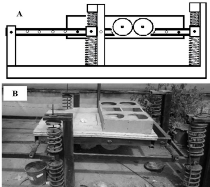
شکل ۱- دستگاه شبیه ساز لرزش. شماتیک (A) و در حال انجام کار (B)
