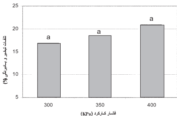
شکل (۳) رابطه فشار کاربرد سیستم با مقدار تلفات تبخیر و بادبردگی
