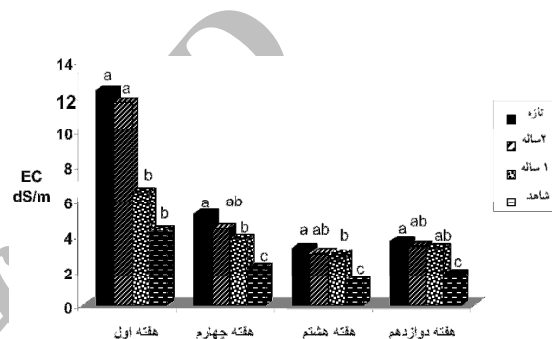
(نمودار ۸) - مقایسه اثر انواع SMC بر تغییرات EC محلول آبشویی خاک
