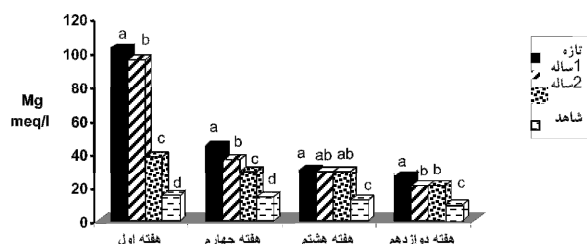
(نمودار ۵) - مقایسه اثر انواع SMC در زمان‌های مختلف در مقدار منیزیم محلول آبشویی خاک
