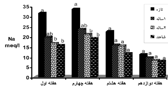
(نمودار ۹) - مقایسه اثر انواع SMC در زمان‌های مختلف در مقدار سدیم محلول آبشویی خاک
