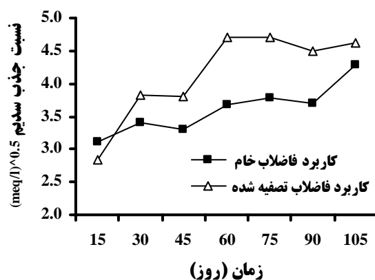
(شکل ۴) - تغییرات میانگین مقدار نسبت جذب سدیوم در زه‌آب خروجی از ستون‌های خاک در طول زمان
