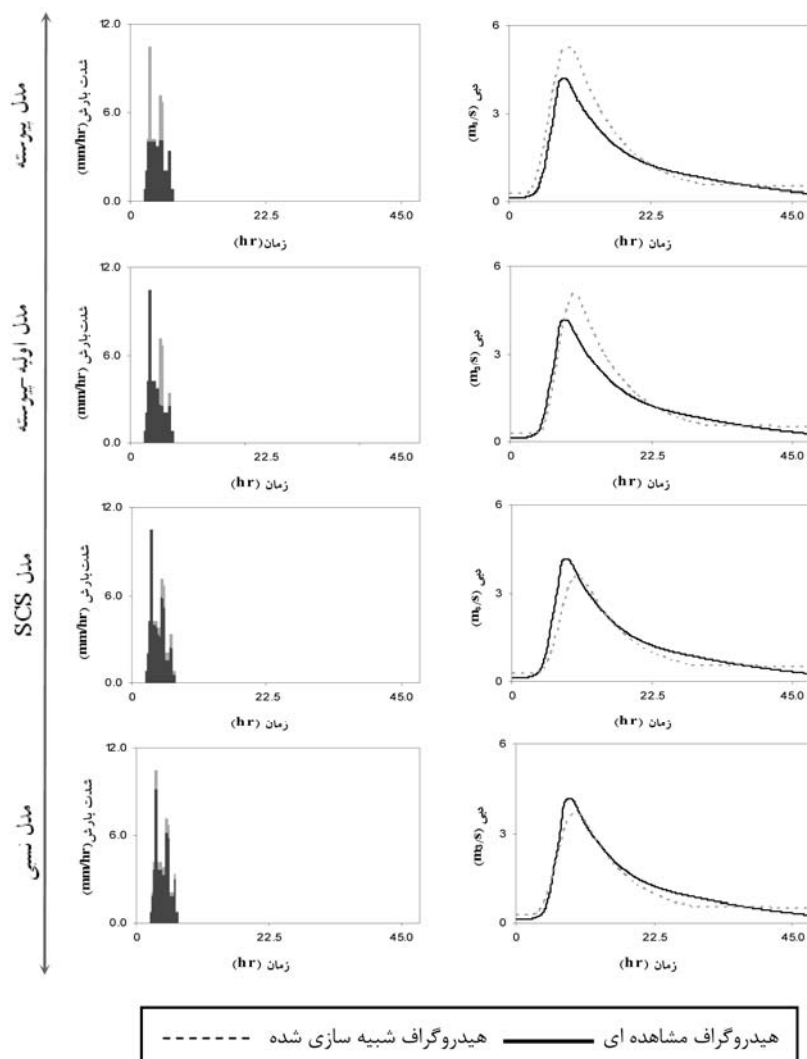
(شکل ۶b) - مقایسه روش‌های تلفات باران در شبیه‌سازی هیدروگراف سیل در مرحله واسنجی (واقع در رگباری ۱۶/۸/۶۶)
