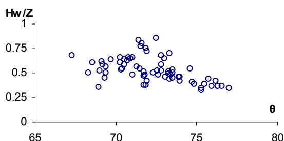
(شکل ۸) - تاثیر H_w/Z بر محل تشکیل عمق بحرانی در سرریز با قطرهای مختلف
