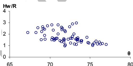
(شکل ۷) - تاثیر H_w/R بر محل تشکیل عمق بحرانی در سرریز با قطرهای مختلف
