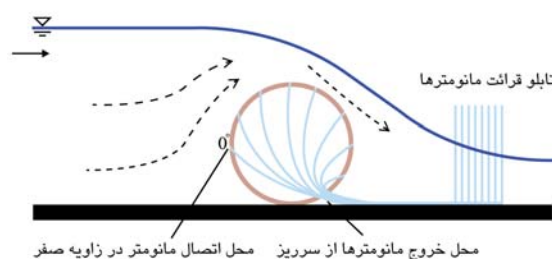
(شکل ۱) - استقرار مانومترها بر روی سرریز در زوایای ۰ تا ۲۱۰ درجه
