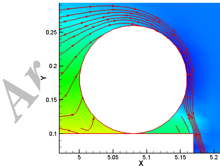
(شکل ۱۵) - خطوط جریان بر روی سرریز استوانه ای و چسبیدگی جریان به سطح سرریز
