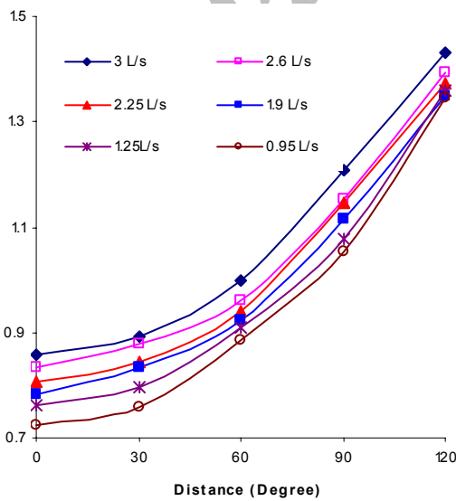
شکل ۵- تغییرات عدد فرود در زوایای مختلف در سرریز با قطر ۶۳ میلیمتر
