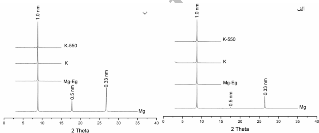
شکل ۳- پراش‌نگاشت پرتو ایکس تیمارهای مختلف بخش رس کانی‌های فلوگوپیت (الف) و موسکویت (ب) مورد استفاده در پژوهش قبل از انجام کشت. K-550 و K، Mg-Eg، Mg به ترتیب نشان دهنده تیمارهای اشباع با منیزیم، منیزیم و اتیلن گلیکول، پتاسیم و پتاسیم و حرارت ۵۵۰ درجه سانتی‌گراد می‌باشند.
