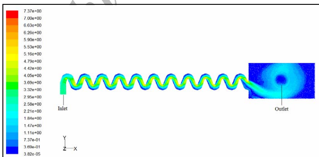
شکل ۱۶- توزیع سرعت جریان در یک واحد قطره چکان A1، حاصل از مدل آسفته تحت فشار ۱۶/۳۳ متر ارتفاع آب
