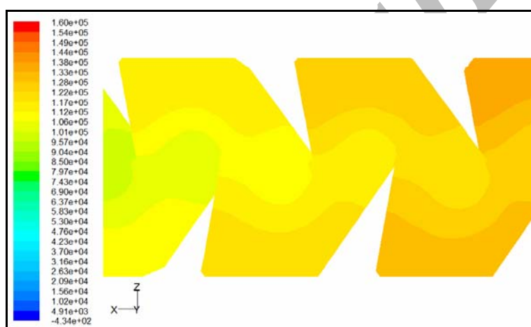
شکل ۱۵- توزیع فشار جریان در یک واحد قطره چکان B، حاصل از مدل آسفته تحت فشار ۱۶/۳۳ متر ارتفاع آب
