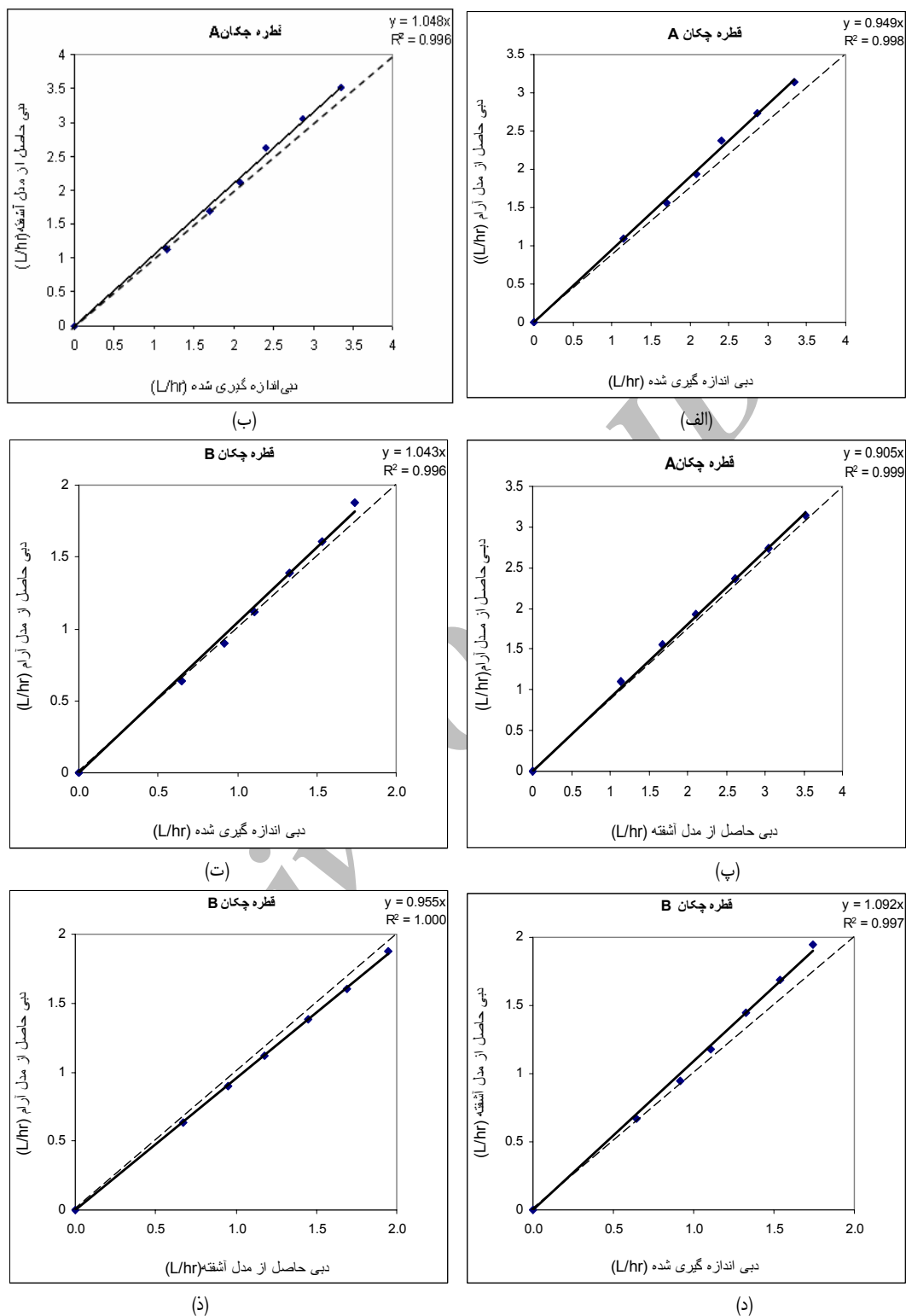
شکل ۲۲- مقایسه دو به دو نتایج حاصل از سه مدل آرام، آشفته و آزمایشگاه برای میانگین نتایج قطره چکان های A1، A2 و A3 با عنوان قطره چکان A و میانگین نتایج سه قطره چکان B1، B2 و B3 با عنوان قطره چکان B
