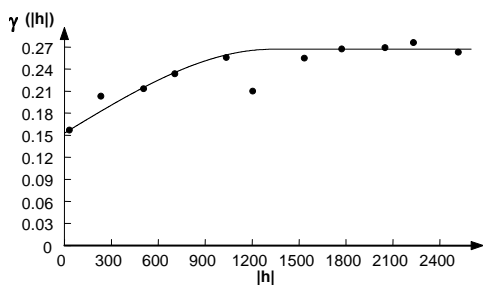
شکل ۲- واریوگرام تجربی و مدل برازش داده شده به داده‌های (A) فراوانی، (B) یکنواختی (C) غنا و (D) تنوع ماکروفون خاک
