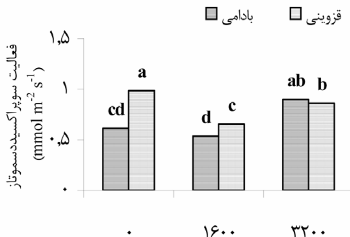
شکل 5- اثر سطوح مختلف شوری و رقم مورد استفاده بر فعالیت آنزیم سوپراکسید سوپرتاز (میلی گرم ملرید سدیم در کیلوگرم خاک)
