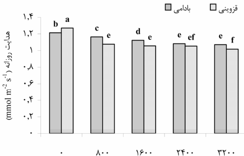
شکل 3- اثر سطوح مختلف شوری بر هدایت روزانه نهال‌های پسته
