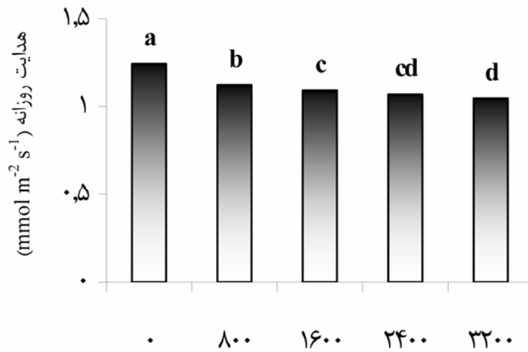
شکل 3- اثر سطوح مختلف شوری بر هدایت روزانه نهال‌های پسته
