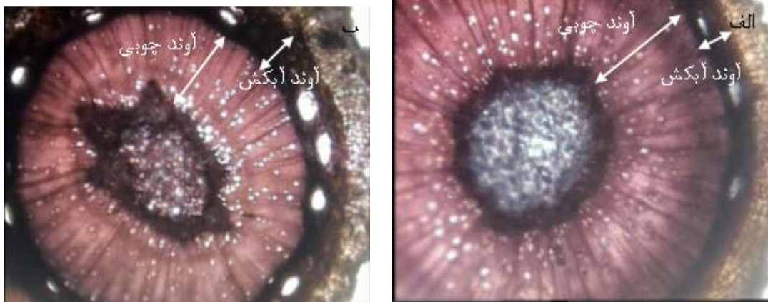
شکل 7- مقایسه ضخامت پارانشیم چوب و قطر آوند آبکش در برش عرضی ساقه تحت شوری 3200 میلی گرم کلریدسدیم در کیلوگرم خاک، عدم کاربرد مس (الف)؛ پس از کاربرد 7/5 میلی گرم مس در کیلوگرم خاک (ب) با بزرگنمایی میکروسکوپ 4x
