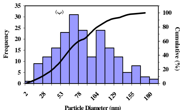
شکل ۲- توزیع فراوانی اندازه نانو ذرات (الف): آهن و (ب): آهن/مس بدست آمده بر اساس اندازه‌گیری قطر ۲۰۰ نانو ذره
