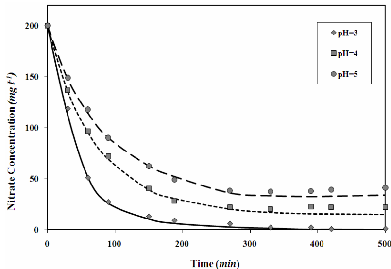
شکل ۴- نتایج حاصل از تأثیر اسیدپتیه محیط واکنش بر احیاء نیترات توسط ذرات Fe/Cu (نقاط) و مدل واکنش جنبشی برازش داده شده (خطوط)
