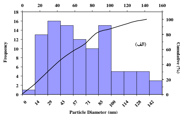
شکل ۲- توزیع فراوانی اندازه نانو ذرات (الف): آهن و (ب): آهن/مس بدست آمده بر اساس اندازه‌گیری قطر ۲۰۰ نانو ذره
