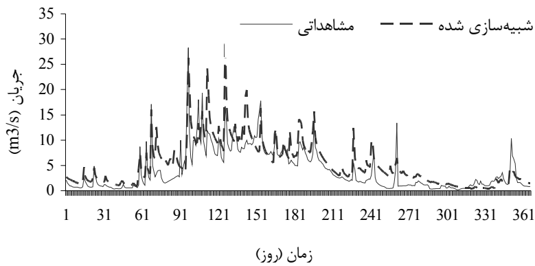
شکل ۹- ارزیابی مدل در سال آبی ۸۴-۱۳۸۳ در حوضه کل کسلیان
