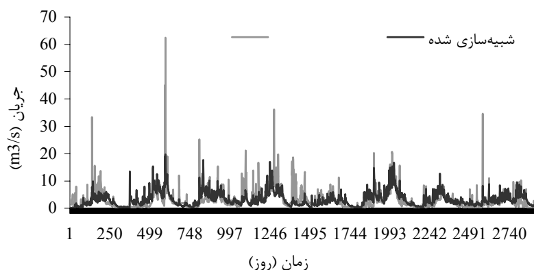
شکل ۶- واسنجی مدل در حوضه کسلیان در طول دوره ۱۳۴۹-۵۷
