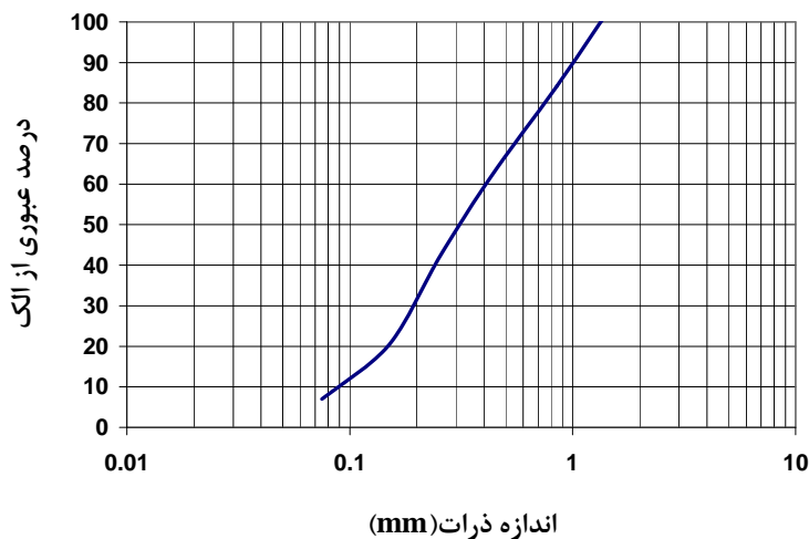
شکل ۲- منحنی دانه‌بندی ماسه‌بادی
