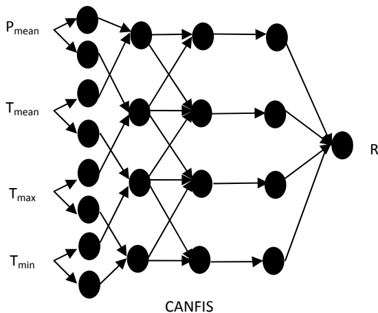
شکل ۲- شماتیکی ساده از شبکه عصبی مصنوعی (ANN) و عصبی-فازی (CANFIS) مورد استفاده
