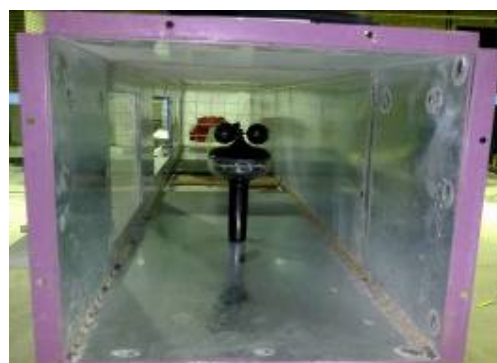
بادسنج پیاله‌ای
