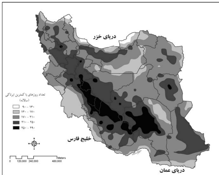
شکل ۶- پهنه بندی سالانه مناطق پرتابش ایران بر اساس میانگین تعداد روزهای با کمترین ابرناکی
