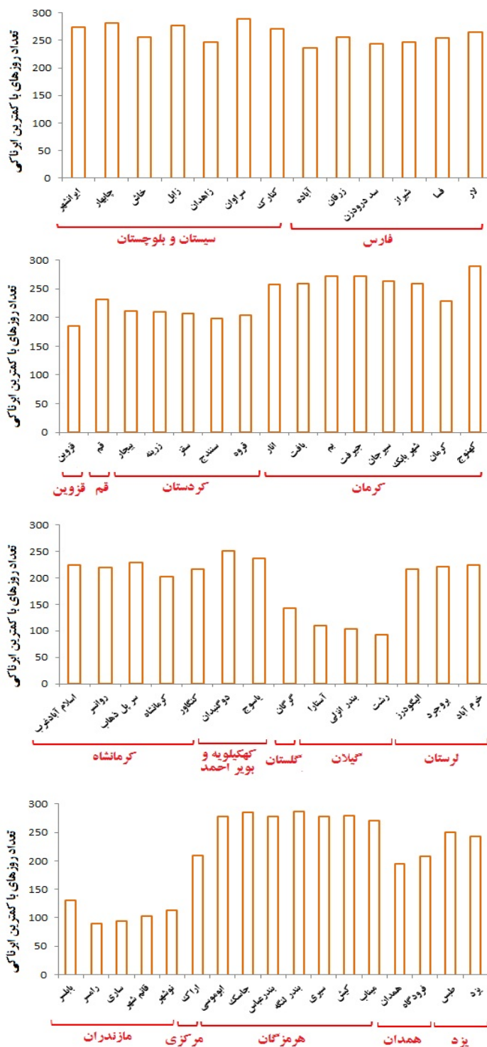
شکل ۲ ب- میانگین سالانه تعداد روزهای با کمترین میزان ابرناکی استان‌های کشور در دوره ۱۳۸۷-۱۳۶۸
