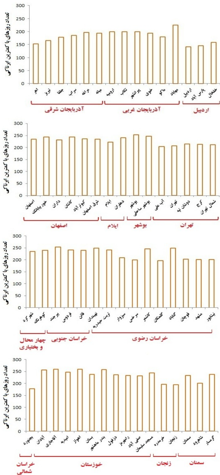
شکل ۲ الف- میانگین سالانه تعداد روزهای با کمترین میزان ابرناکی استان‌های کشور در دوره ۱۳۸۷-۱۳۶۸
