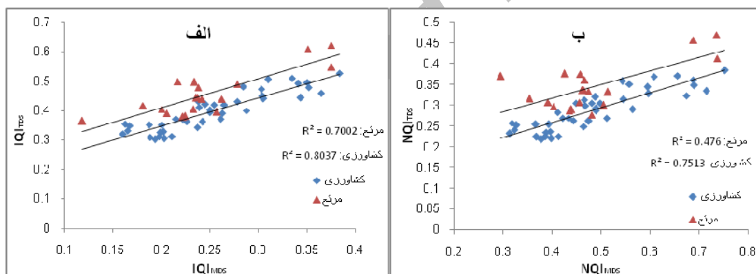
شکل ۱- رابطه خطی الف) IQI MDS و IQI TDS ب) NQI MDS و NQI TDS در نمونه خاک‌های زمین‌های کشاورزی و مرتع
