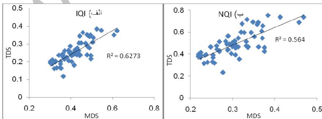
شکل ۲- رابطه خطی الف) IQI MDS و IQI TDS ب) NQI MDS و NQI TDS در کل نمونه خاک‌ها
