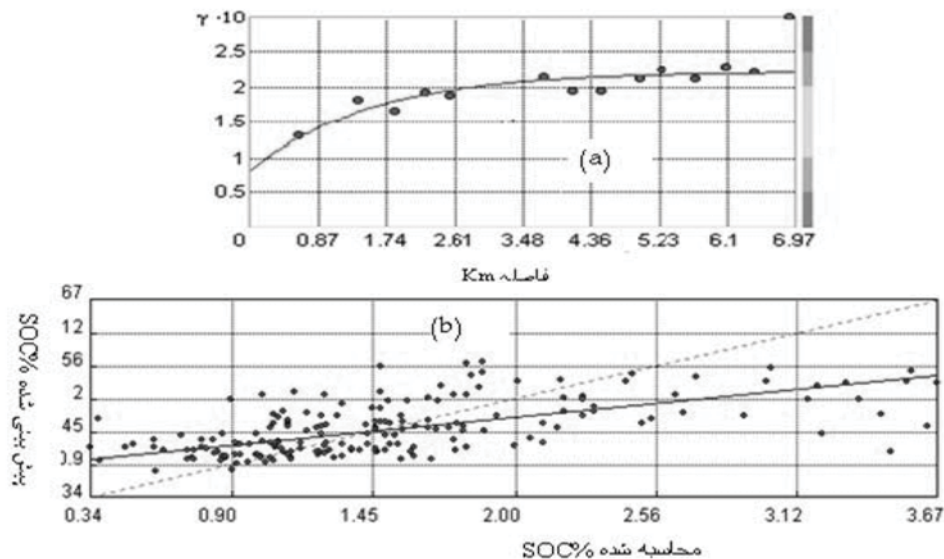
شکل ۲- مشخصات نیم تغییرنا (a) و نمودار پخشیه مقادیر برآوردی در مقابل مقادیر اندازه گیری شده (b) در روش درون یابی کریجینگ معمولی برای داده‌های کربن آلی خاک در کل حوزه
