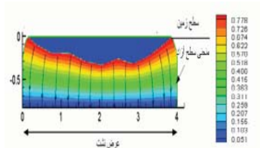
شکل ۵ - خطوط جریان و پتانسیل و عرض نشت نهر شیخ سرمست
