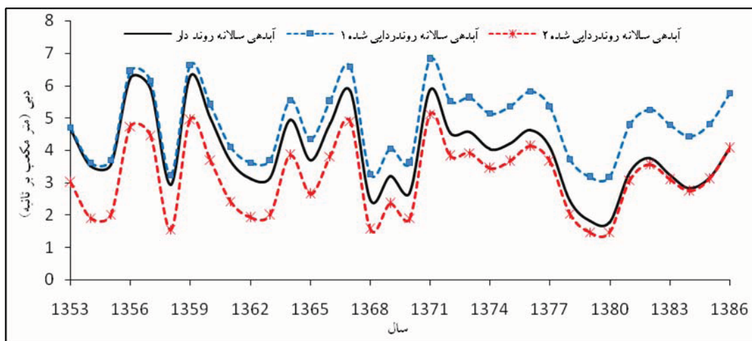
شکل ۳- سری‌های زمانی آبدهی سالانه رونددار و روندزدایی شده به منظور مدیریت بالا دست و پایین دست، ایستگاه تاز کند
