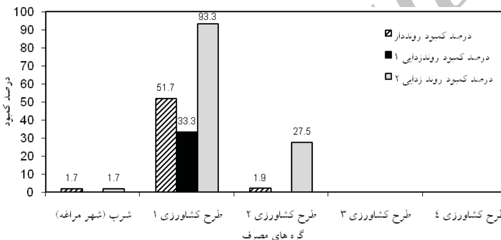
شکل ۵- مقادیر درصد کمبود سالانه در گره‌های مصرف به تفکیک سری‌های زمانی رونددار و رونزدایی شده ۱ و ۲
