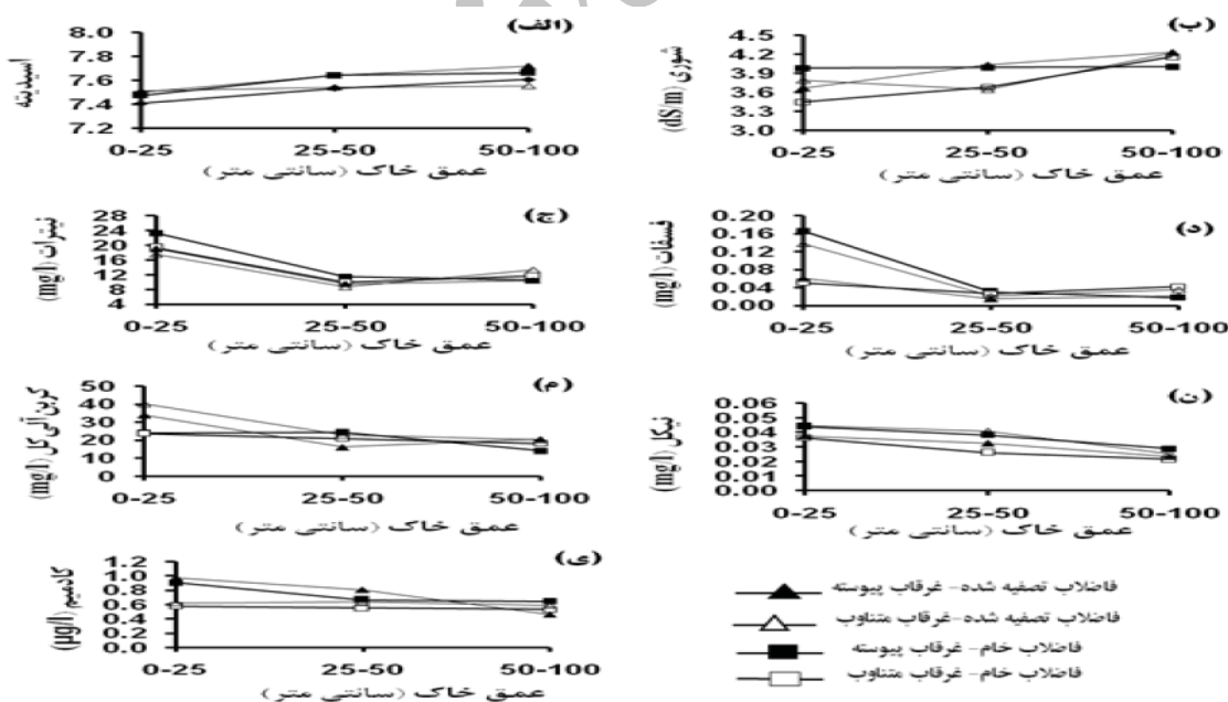
شکل ۴- تأثیر عبور فاضلاب‌ها از ستون‌های خاک بر مقدار برخی پارامترهای شیمیایی در اعماق مختلف خاک
