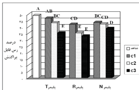
شکل ۱۱- اثر تیمارهای پلیمر بر میزان رس قابل پراکنش خاک لومرسی سiltی
