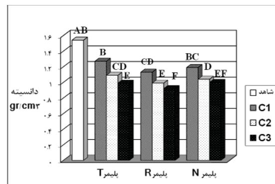
شکل ۱۲- اثر تیمارهای پلیمر بر چگالی توده خاک شن لومی
