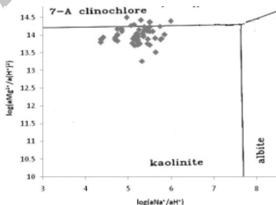
شکل ۴- نمودارهای \text{Log}(a\text{Ca}^{2+}/a(\text{H}^+)^2) و \text{Log}(a\text{Mg}^{2+}/a(\text{H}^+)^2) در مقابل \text{Log}(a\text{Na}^+/a(\text{H}^+)) در رودخانه کارده
