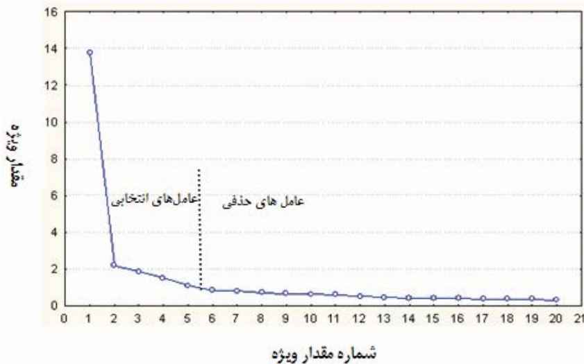
شکل ۱- نمودار صخره‌ای حاصل از تجزیه به عامل‌های مقادیر SPI سه ماهه حوضه دریاچه ارومیه
