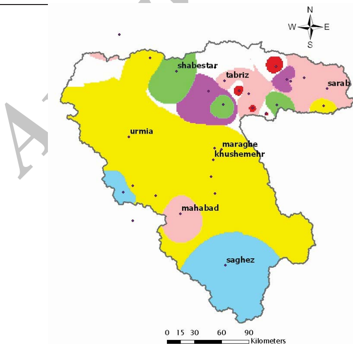
شکل ۳- نقشه همگنی نواحی بدست آمده از تجزیه به عامل‌ها برای داده‌های SPI دوازده ماهه
