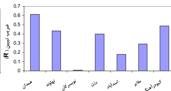
شکل ۶- مقایسه همبستگی آماری عملکرد با کمبود بارش مرجع در شهرهای مورد مطالعه برای گندم آبی و گندم دیم
