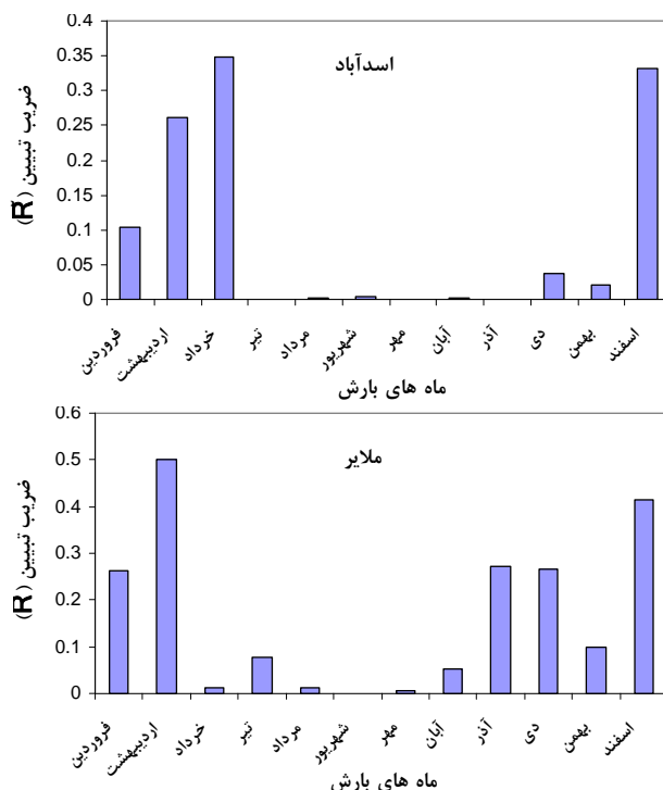
شکل ۳- مقایسه ضرایب تبیین روابط رگرسیونی بین عملکرد گندم دیم با ماه‌های بارش در مجموعه شهرهای استان همدان
