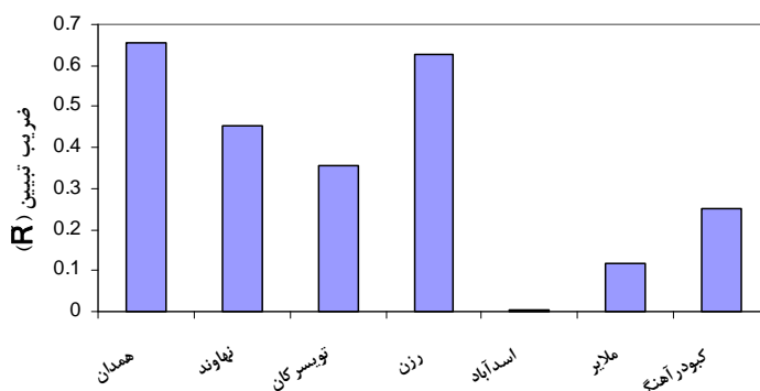
شکل ۵- توزیع پراکندگی ضرایب تبیین روابط رگرسیونی شاخص عملکرد سالیانه گندم با بارش سالیانه در مجموعه ایستگاه‌های استان همدان
