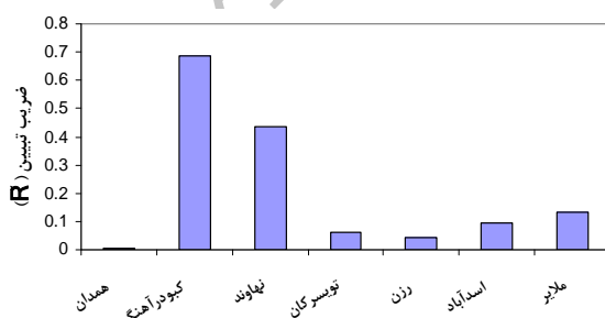
شکل ۶- مقایسه همبستگی آماری عملکرد با کمبود بارش مرجع در شهرهای مورد مطالعه برای گندم آبی و گندم دیم
